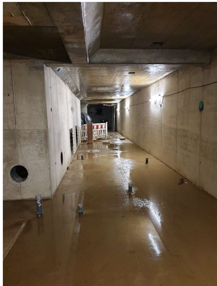
Bereich unterhalb des Schwimmerbeckens - Seitenwand Becken
